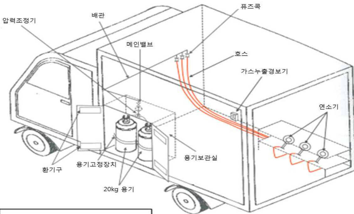
<표 1> 이동용 음식판매 화물자동차 LPG사용시설 표준설치 예시
