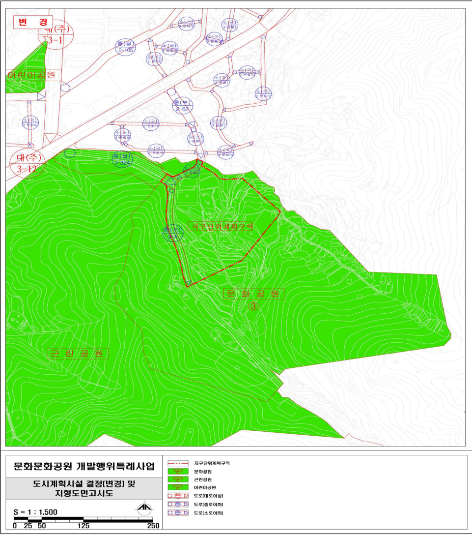
< 도시계획시설 결정(변경)도 - 변경 >
